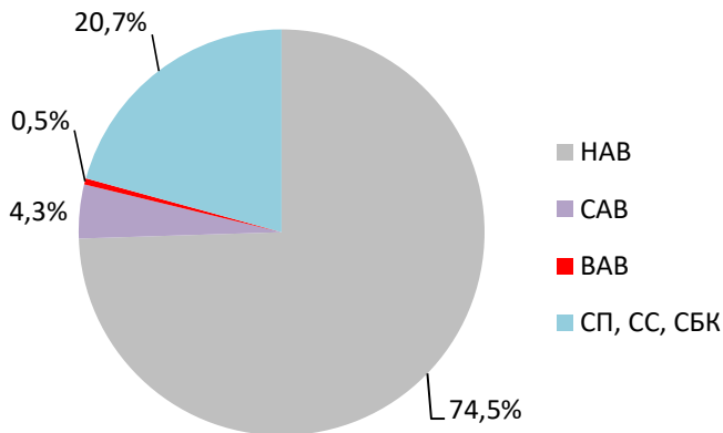
Розподіл об'ємів накопичених ТРВ на АЕС (з урахуванням СП, СС (ПАЕС) та СБК (РАЕС))
