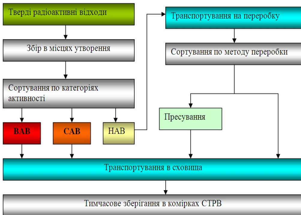
Схема поводження з ТРВ на ПАЕС
